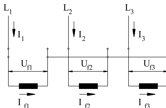
Figura 1.8a - Ligações
