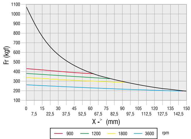
Carcaça 160
