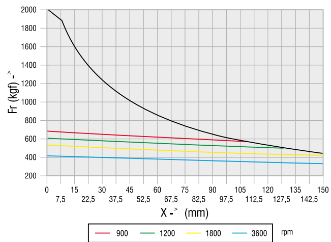
Carcaça 200
