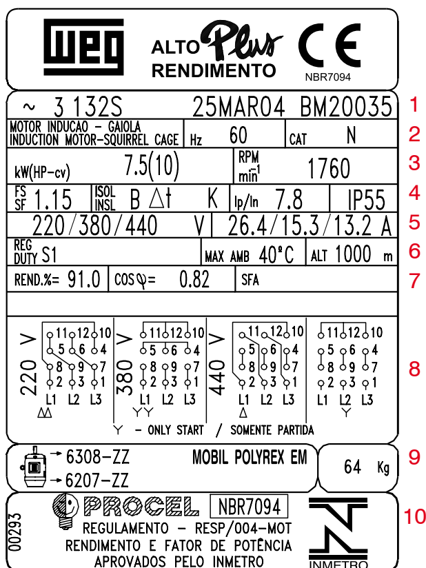
Figura 17.1 - Placa de identificação
