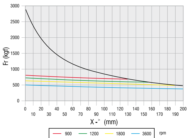
Carcaça 250
