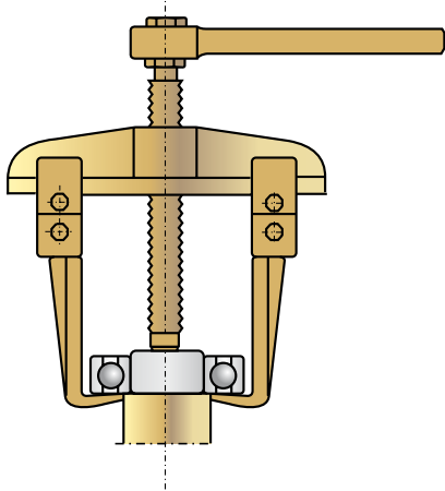
Figura 15.1 - Extrator de rolamentos
