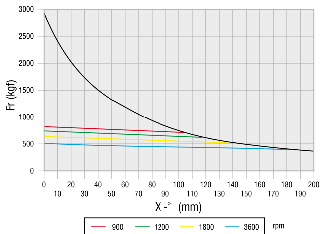
Carcaça 225
