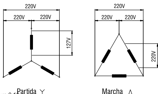
Figura 2.12 Partida Y
