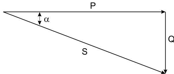
Figura 1.2 - Triângulo de potências (carga indutiva)
