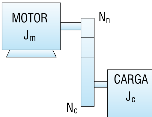
Figura 3.3 - Momento de inércia em rotações diferentes
