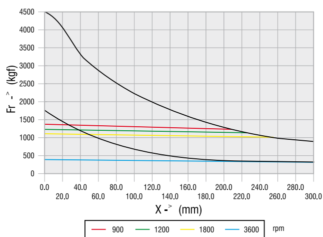
Carcaça 355
